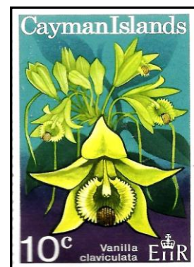
Vanilla claviculata
